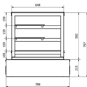
VISTA LATERAL
