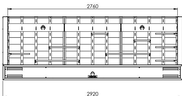
Vue frontale
