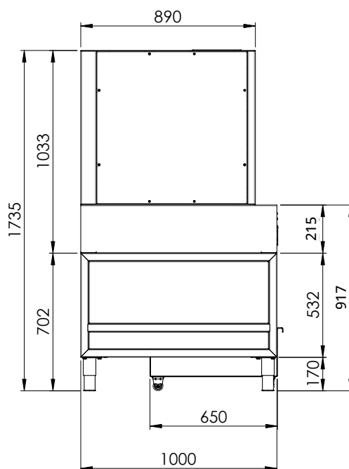
VUE LATÉRALE
