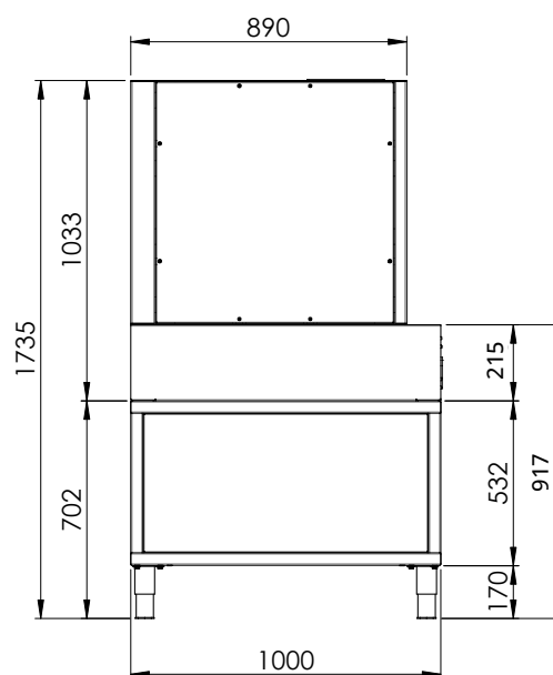
VUE LATÉRALE
