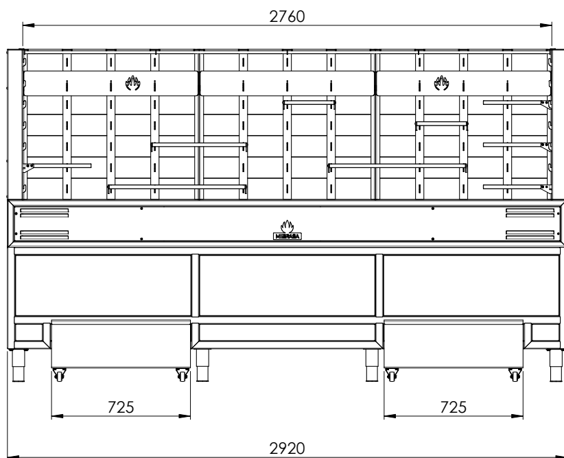
VUE FRONTALE
