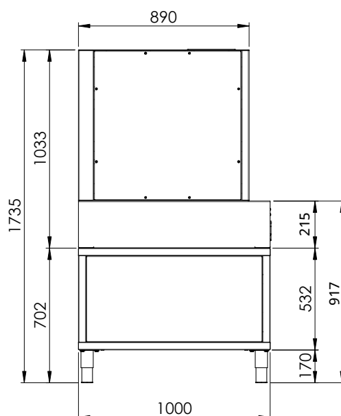
VUE LATÉRALE
