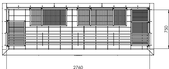
Vue supérieure
