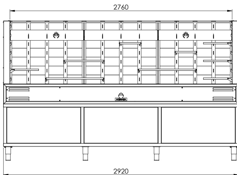
VUE FRONTALE
