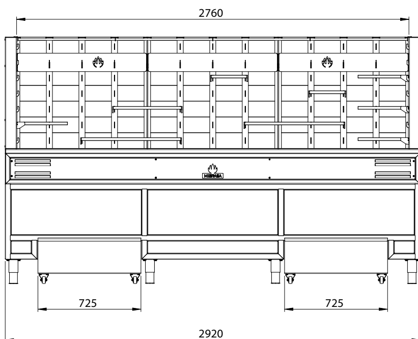
VUE FRONTALE
