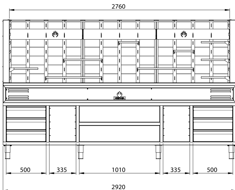
VUE FRONTALE
