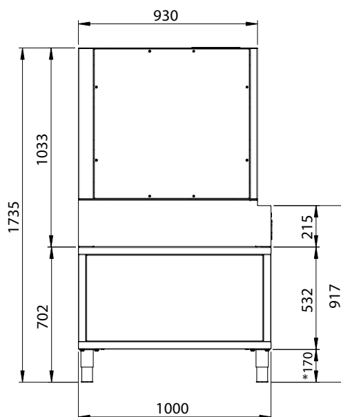
VUE LATÉRALE
