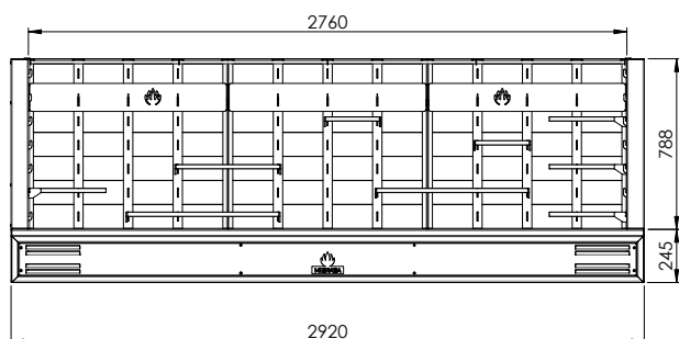
Vue frontale
