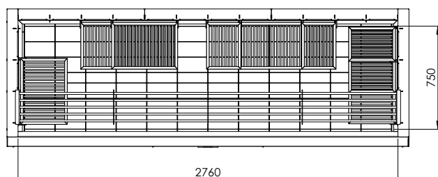
Vue supérieure
