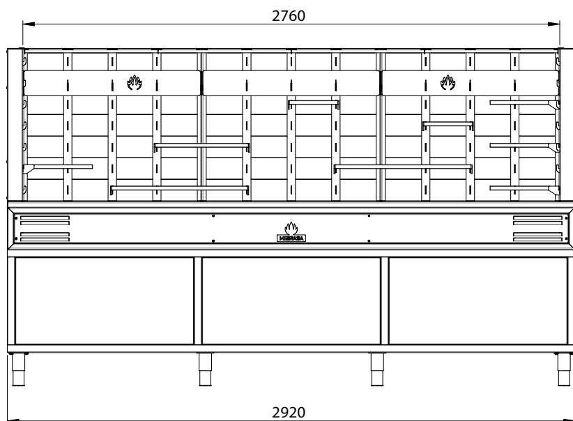
VUE FRONTALE
