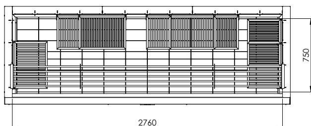
Vista superiore
