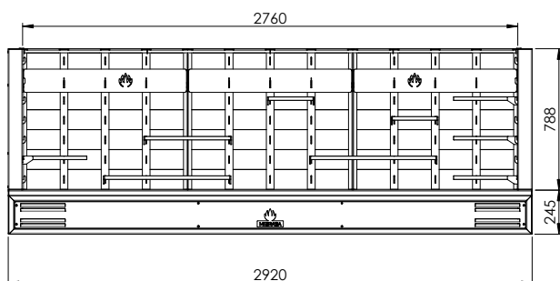
Vista frontale
