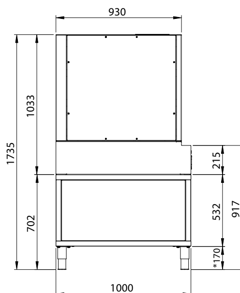
VISTA LATERALE
