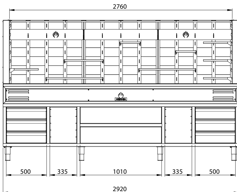
VISTA FRONTALE
