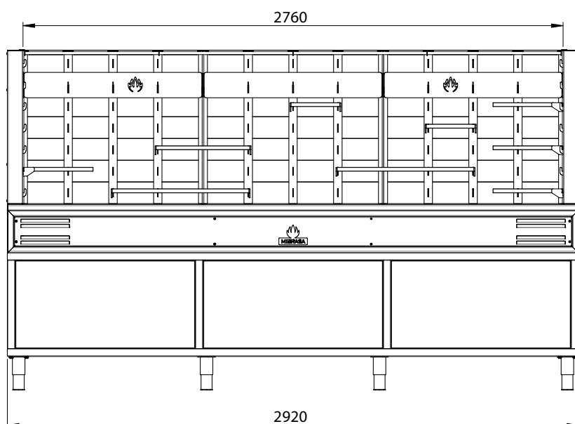
VISTA FRONTALE
