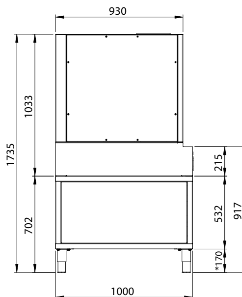
VISTA LATERALE
