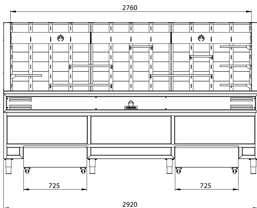
VISTA FRONTALE
