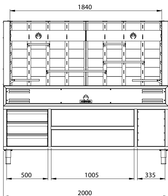
VUE FRONTALE
