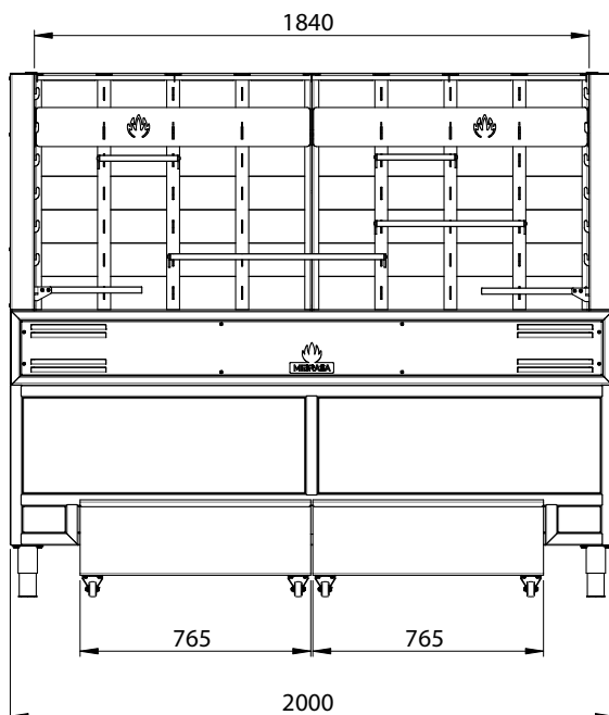
VUE FRONTALE
