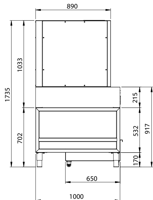
VUE LATÉRALE
