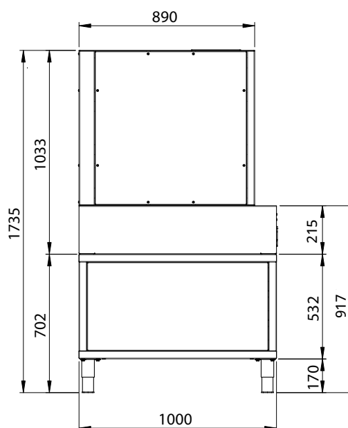
VUE LATÉRALE
