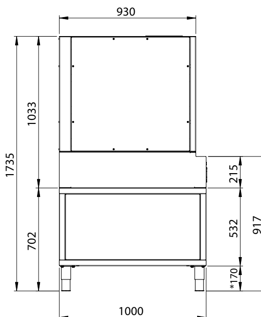
VISTA LATERAL
