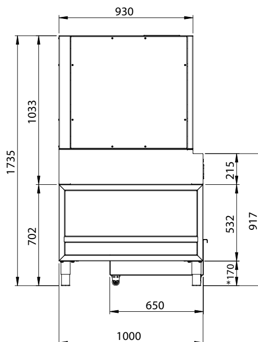
VISTA LATERAL
