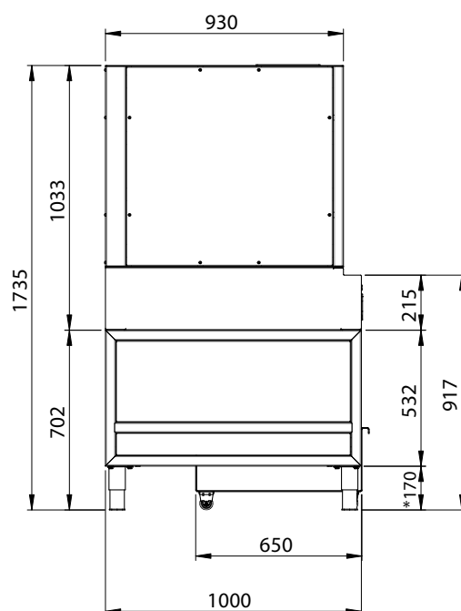
VUE LATÉRALE
