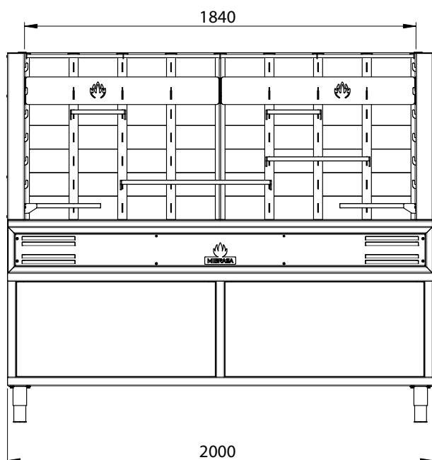
VUE FRONTALE
