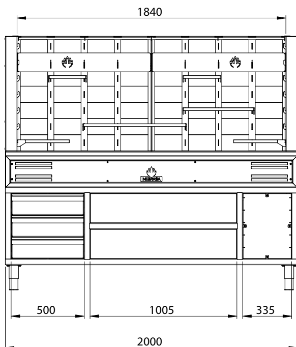
VUE FRONTALE
