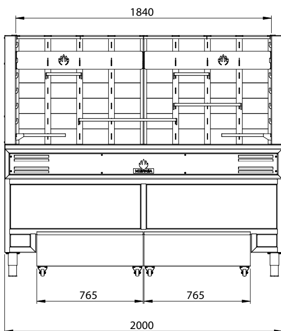
VUE FRONTALE
