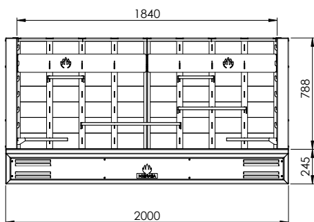
Vue frontale
