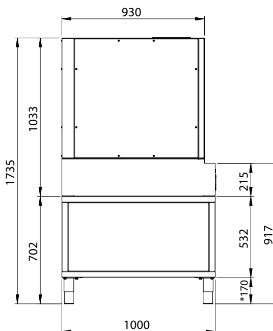
VISTA LATERALE
