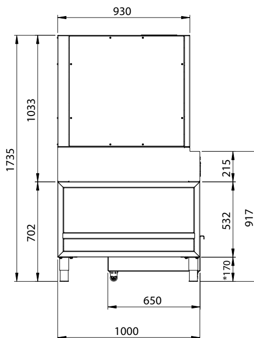
VISTA LATERALE
