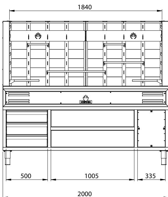
VISTA FRONTALE
