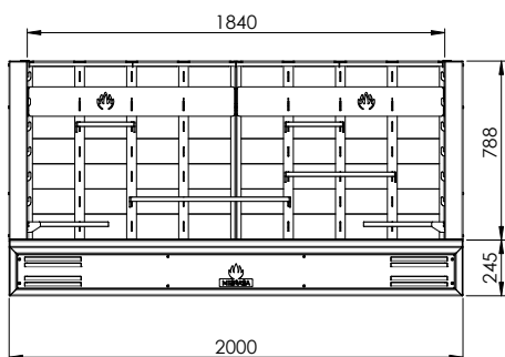
Vista frontale
