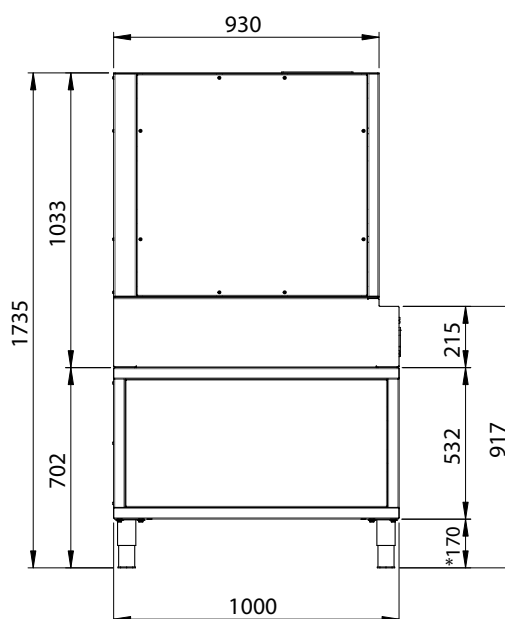
VISTA LATERALE
