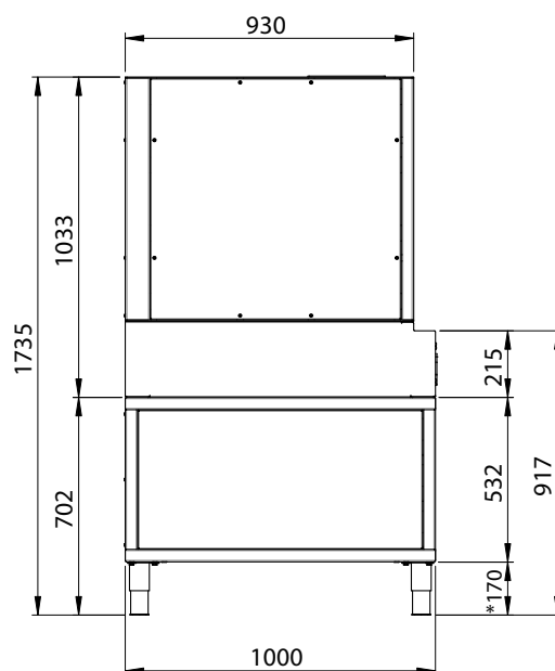
VISTA LATERAL
