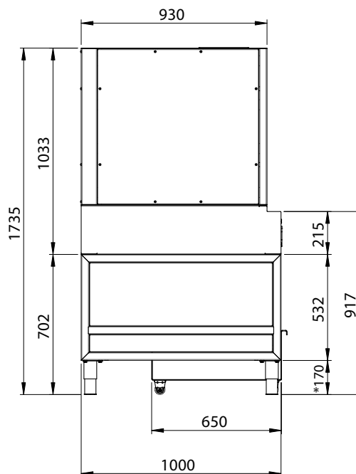
VISTA LATERAL
