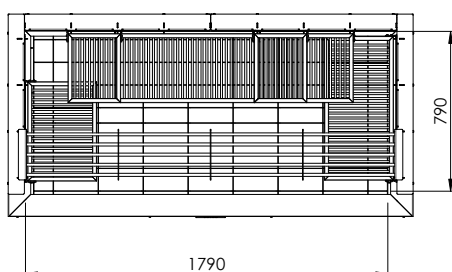
Vista superiore
