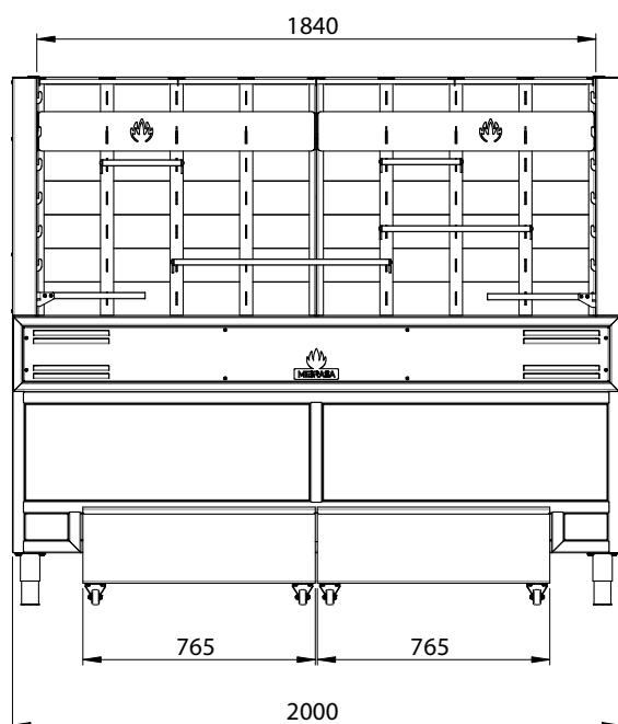
VISTA FRONTALE
