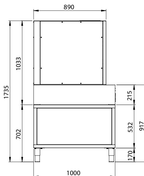
VISTA LATERALE
