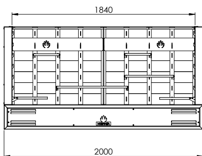
Vista frontale
