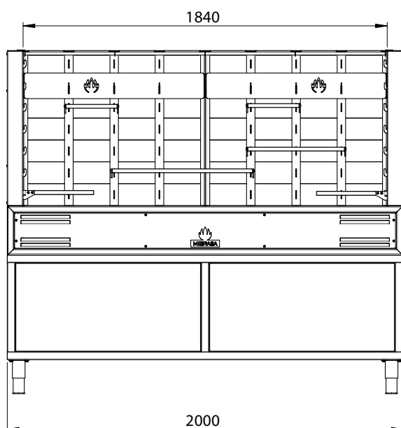
VISTA FRONTALE
