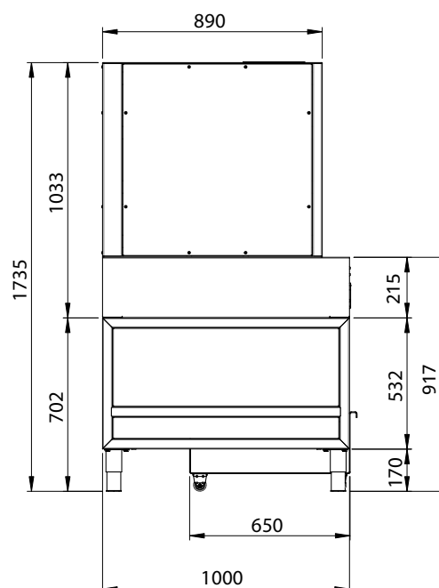
VISTA LATERALE
