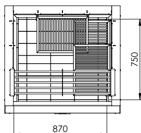
Vista superior
