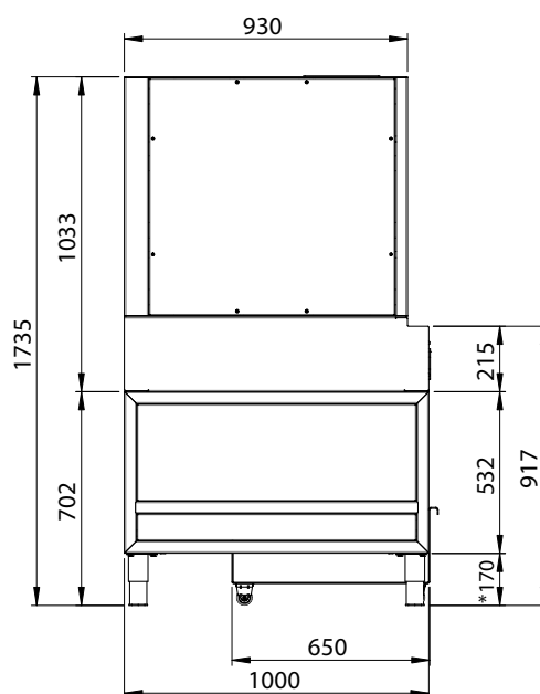
VISTA LATERALE
