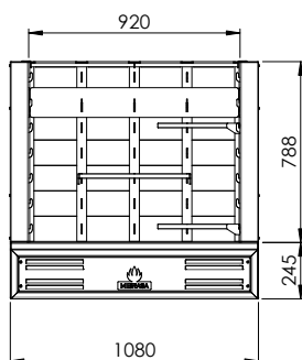
Vista frontale
