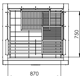
Vista superiore
