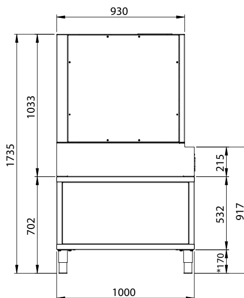
VISTA LATERALE
