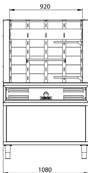
VISTA FRONTALE
