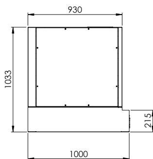
Vista laterale
