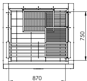
Vista superior
