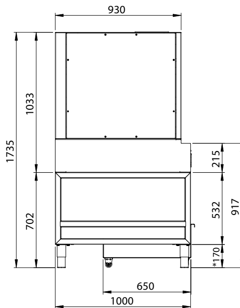
VISTA LATERAL
