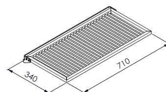
Parrilla grande [CPS-71]
