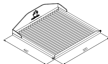
DIMENSIONES DEL SOPORTE BANDEJA
