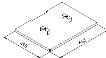
DIMENSIÓN TAPA (OPCIONAL)
