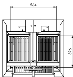
Vue supérieure
