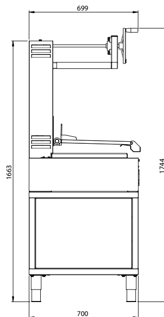
VUE LATÉRALE
