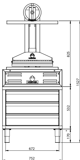
VUE FRONTALE
