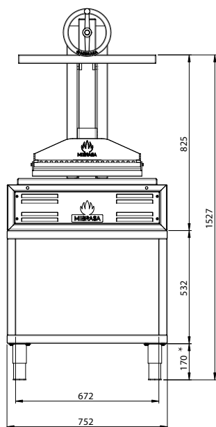
VUE FRONTALE
