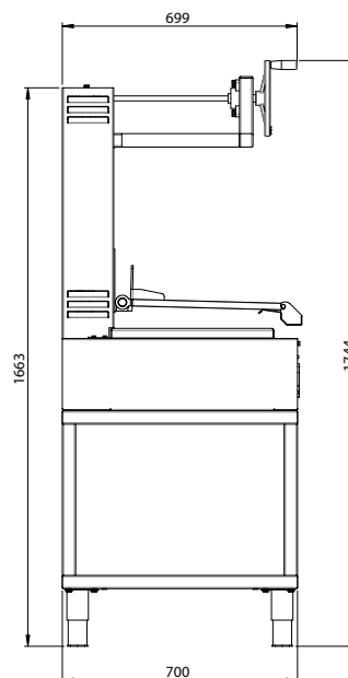
VUE LATÉRALE
