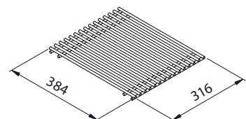
Mediana (x6)
