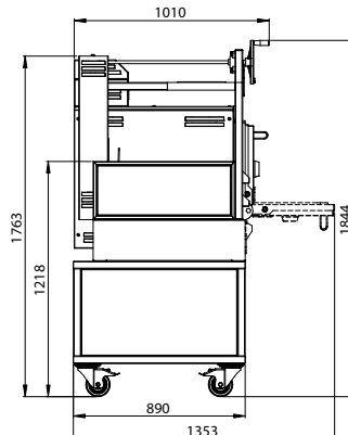
Vista laterale
