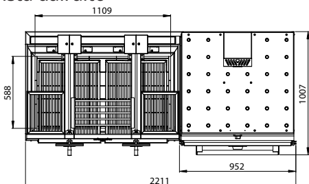
Vista dall'alto
