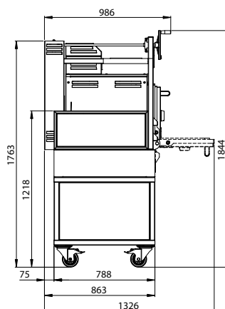
Vista laterale
