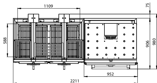
Vista dall'alto
