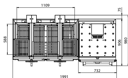
Vista dall'alto
