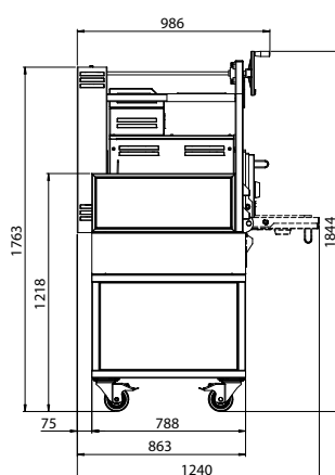
Vista laterale
