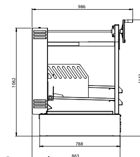
Graella en V
