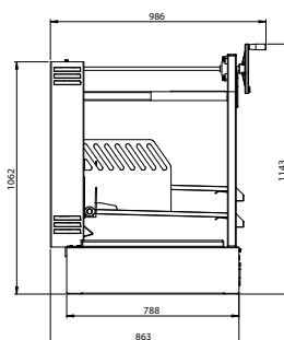
Brûleur
