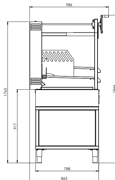
VUE LATÉRALE
