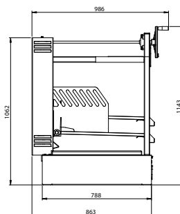
Brûleur
