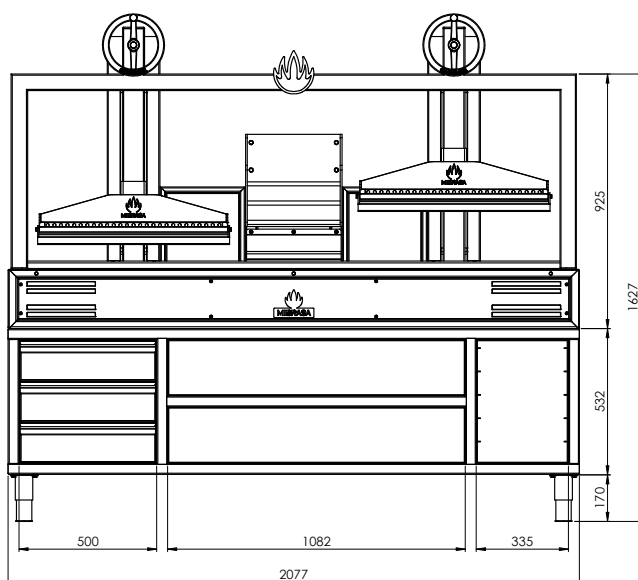
VUE FRONTALE
