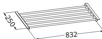
DIMENSIONS DEL SUPORT DE COCCIÓ VERTICAL
