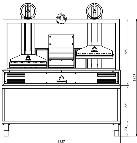
VUE FRONTALE
