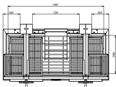
Vue supérieure
