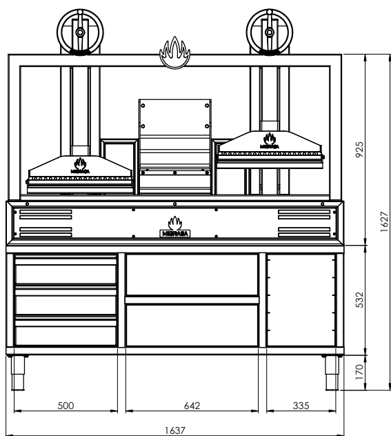
VUE FRONTALE
