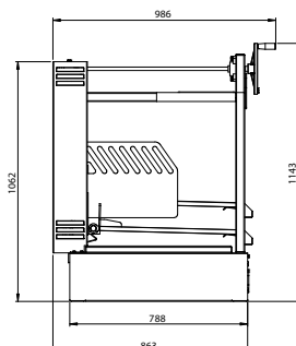
Vue latérale
