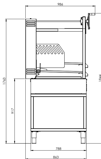
VUE LATÉRALE
