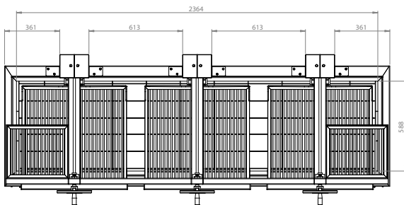
Vista dall'alto
