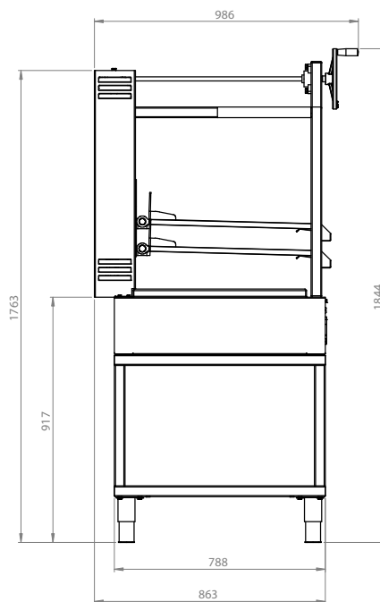
VISTA LATERALE
