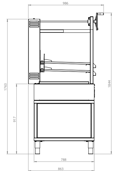
VISTA LATERALE
