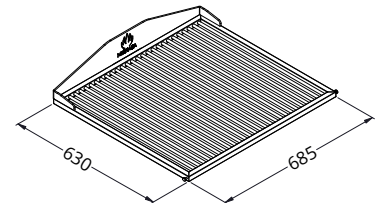
DIMENSIONI SUPPORTO VASSOIO
