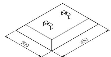
DIMENSIONI COPERCHIO INOX OPZIONALE
