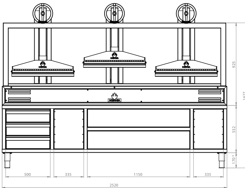
VISTA FRONTALE
