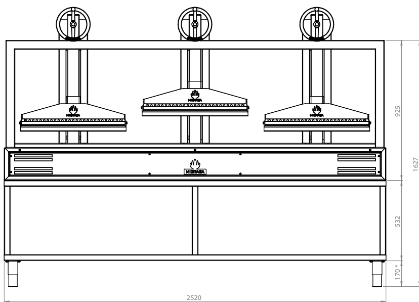
VISTA FRONTALE
