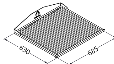
DIMENSIONS DE LA GRAELLA
