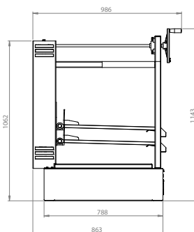
Grille ronde
