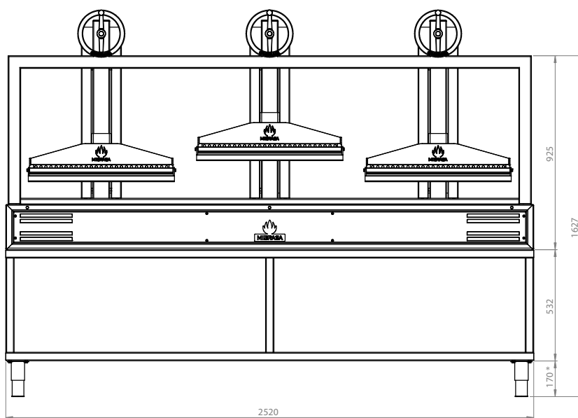
VUE FRONTALE
