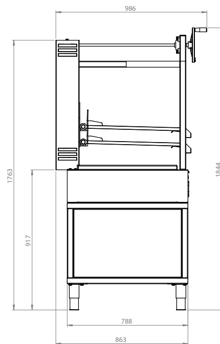
VUE LATÉRALE
