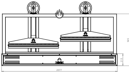
Vue frontale
