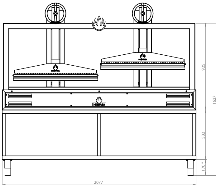
Vue frontale
