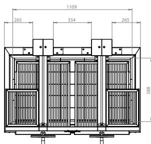
Vue supérieure
