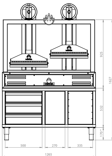
VUE FRONTALE
