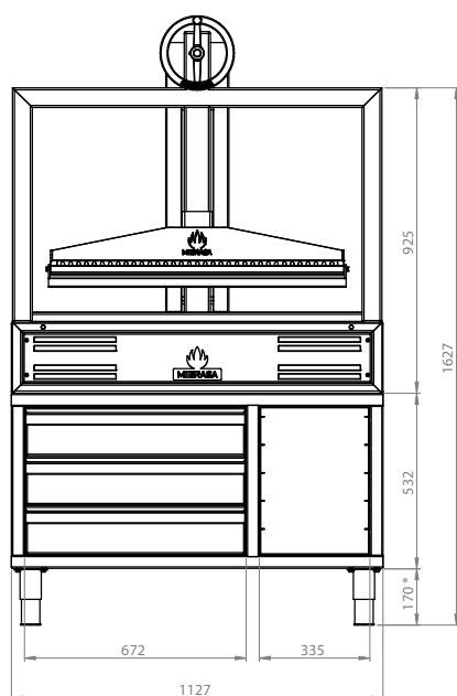
VUE FRONTALE
