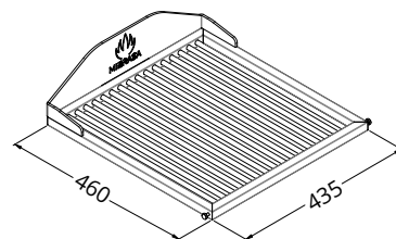
DIMENSIONI SUPPORTO VASSOIO
