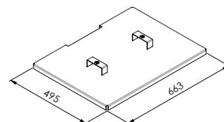
DIMENSIONI COPERCHIO INOX OPZIONALE
