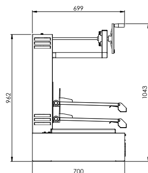
Vista lateral
