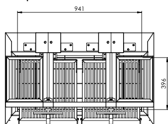
Vista superior
