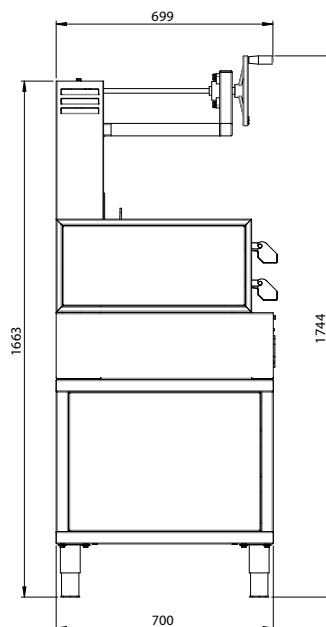
VUE LATÉRALE
