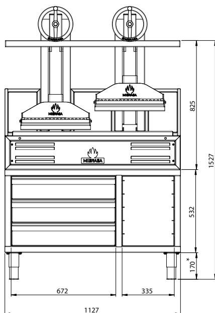
VUE FRONTALE
