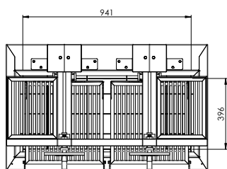
Vue supérieure
