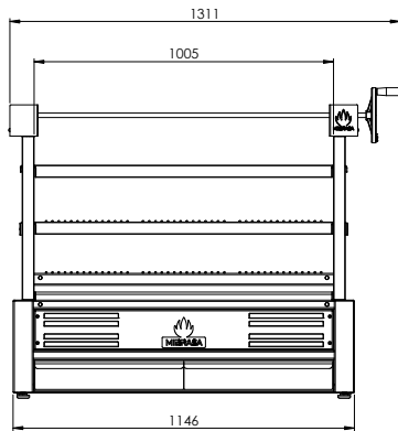
Vista frontale
