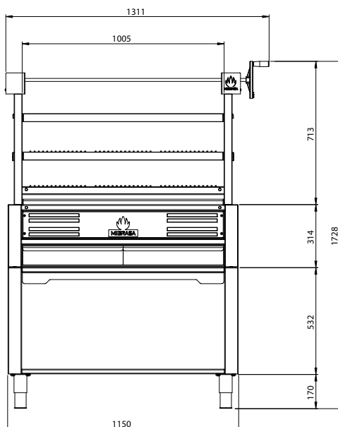
VISTA FRONTALE
