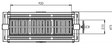
Vista dall'alto
