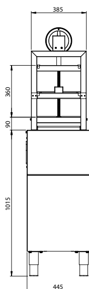
VISTA LATERAL
