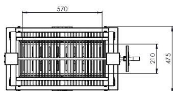
Vista superior
