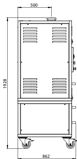
Vista laterale
