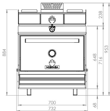
Vista frontale
