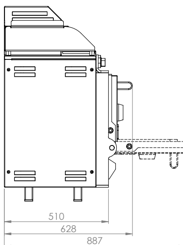
Vista laterale
