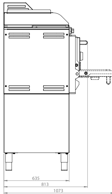
Vista lateral
