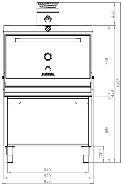
Vue frontale
