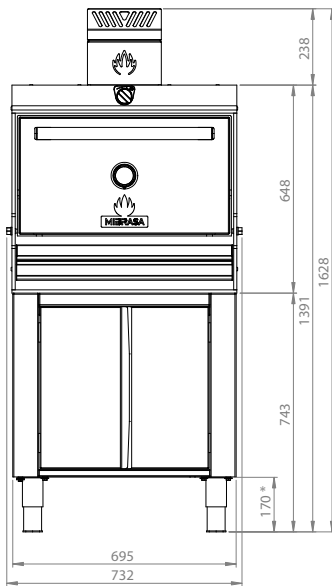
Vista frontale
