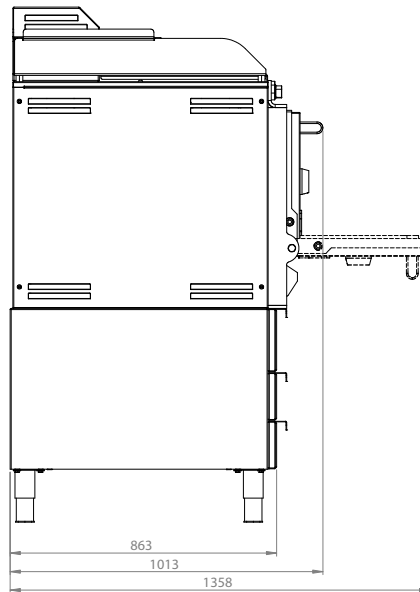
Vista laterale
